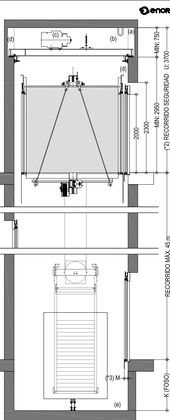
SECCIÓN E.1/60
