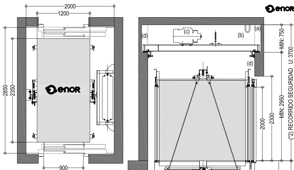
PLANTA GENERAL E.1/50
