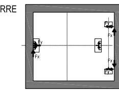
ESQUEMA CARGAS ESTRUCTURALES (KN) EN TESTERO, FOSO y CIERRE.
