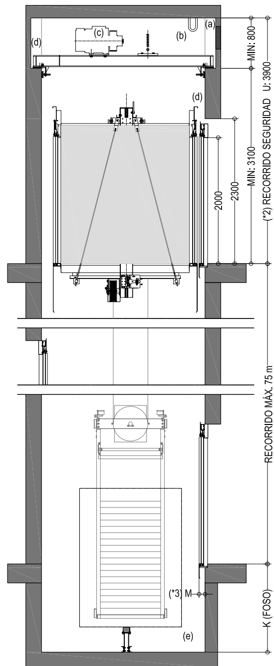
SECCIÓN E.1/60
