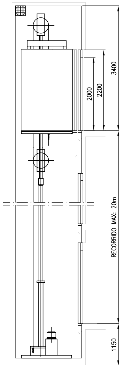
SECCION VERTICAL 1/60
