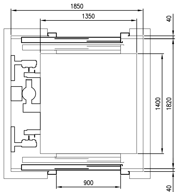
PLANTA GENERAL 1/30
