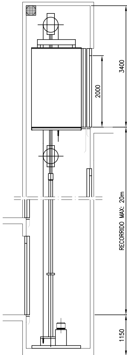
SECCION VERTICAL 1/60
