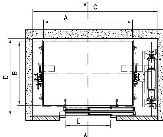
PLANTA GENERAL (E:1/60)
