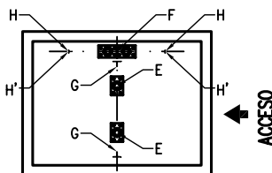
CARGAS EN EL FOSO
