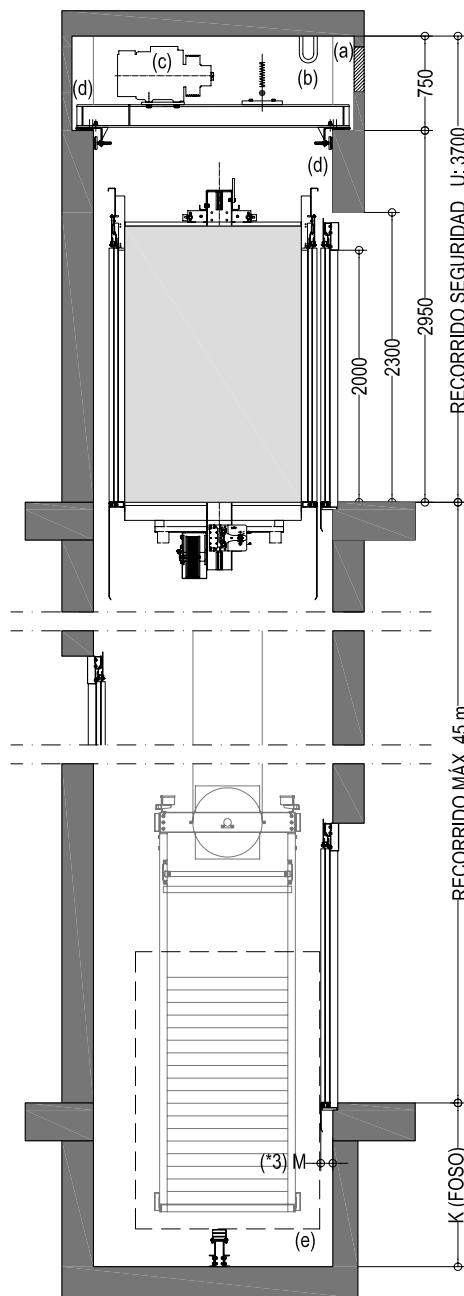
SECCIÓN E.1/60
