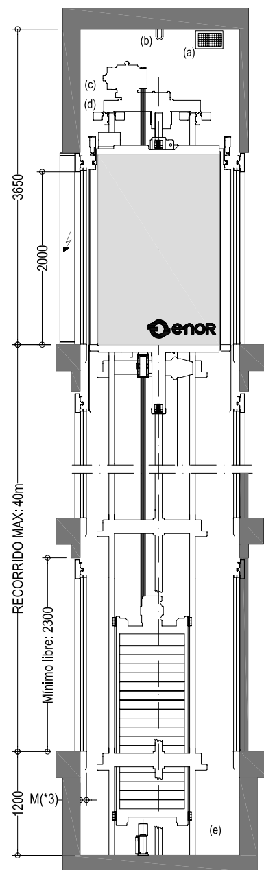
SECCIÓN E.1/60
