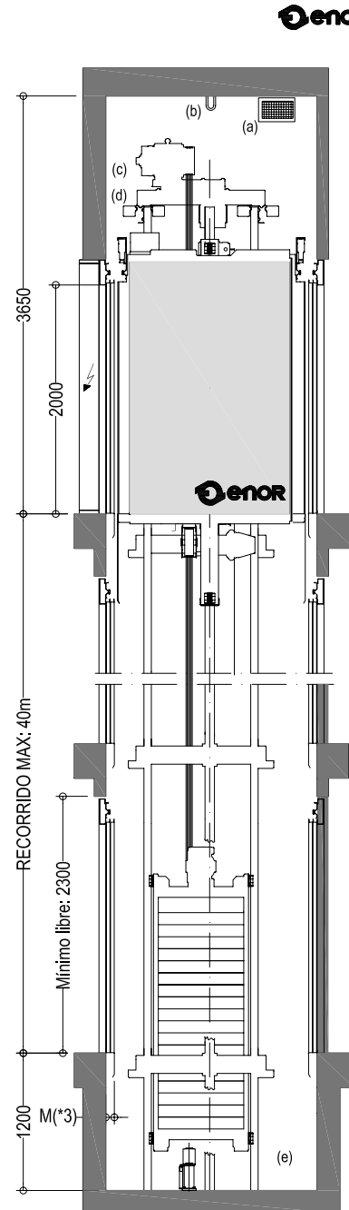
SECCIÓN E.1/60
