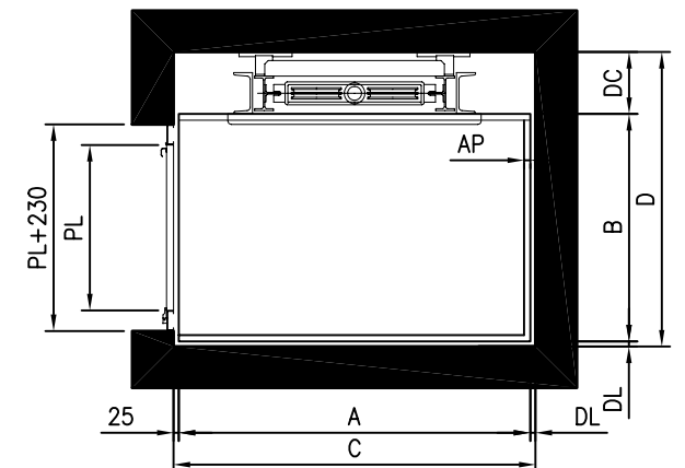
Disposición 2 - 3, simple embarque lateral.
