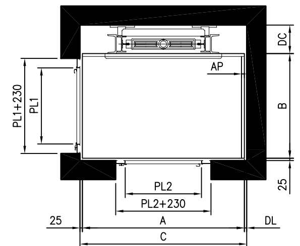
Disposición 5 - 6, doble embarque 90°. NOTA: Disposición no disponible para Cabina.
