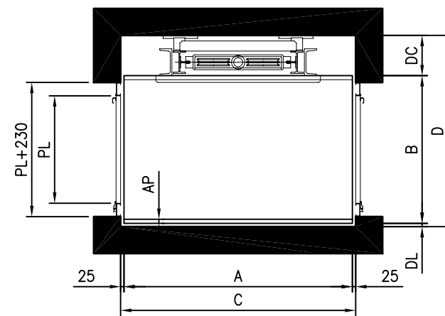
Disposición 4, doble embarque 180°.
