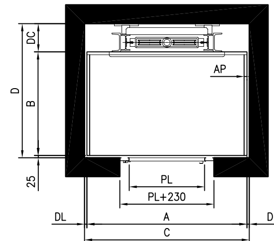
Disposición 1, simple embarque frontal.
