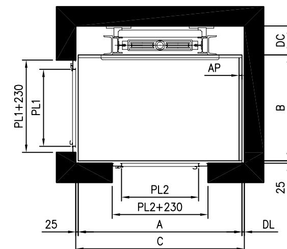
Disposición 5 - 6, doble embarque 90°. NOTA: Disposición no disponible para cabina.
