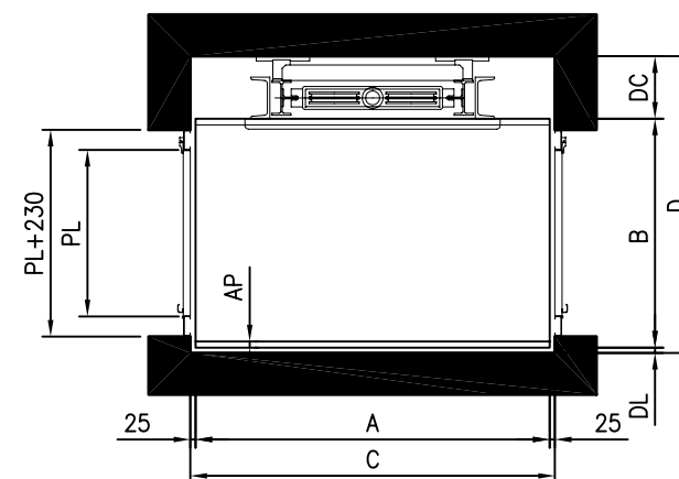
Disposición 1, simple embarque frontal.
