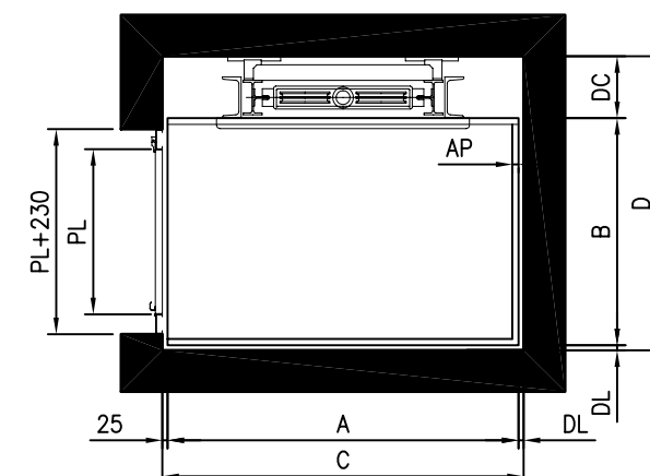
Disposición 2 - 3, simple embarque lateral.
