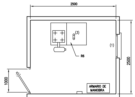
PLANTA GENERAL
