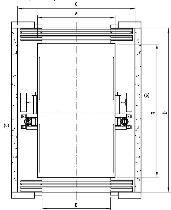
PLANTA GENERAL
