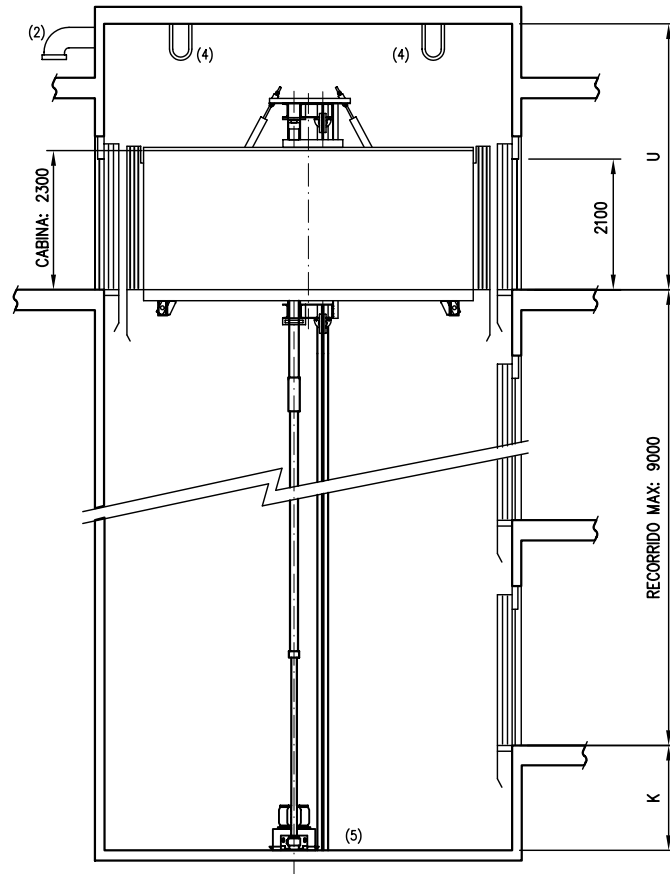
SECCIÓN VERTICAL
