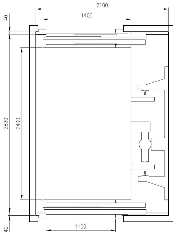
PLANTA GENERAL 1/30
