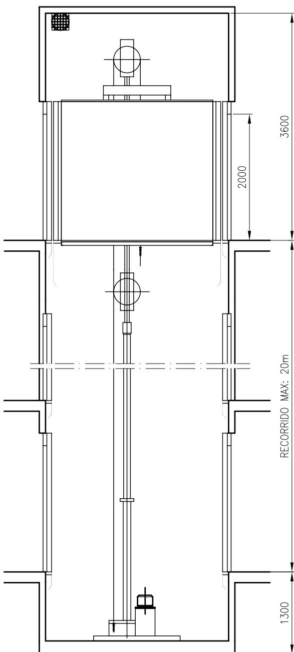
SECCION VERTICAL 1/60
