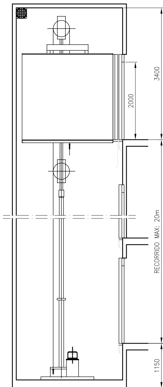
SECCION VERTICAL 1/60
