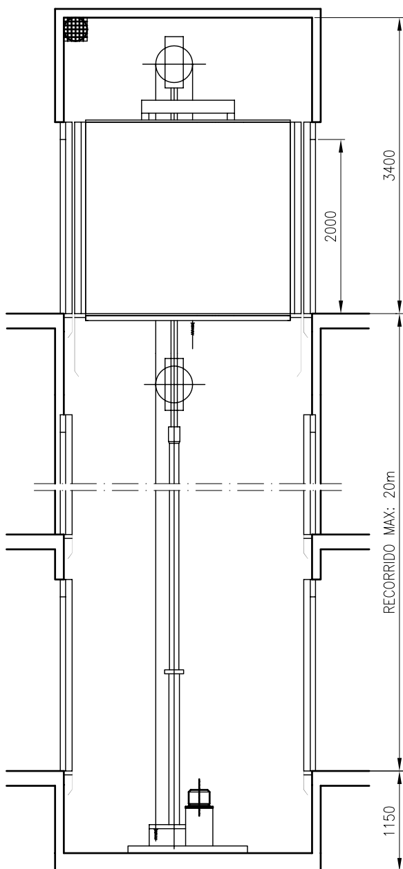
SECCION VERTICAL 1/60
