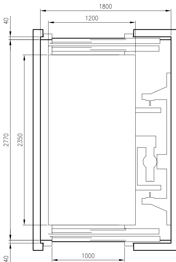
PLANTA GENERAL 1/30
