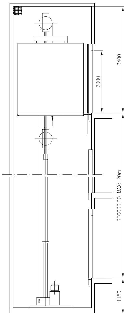
SECCION VERTICAL 1/60
