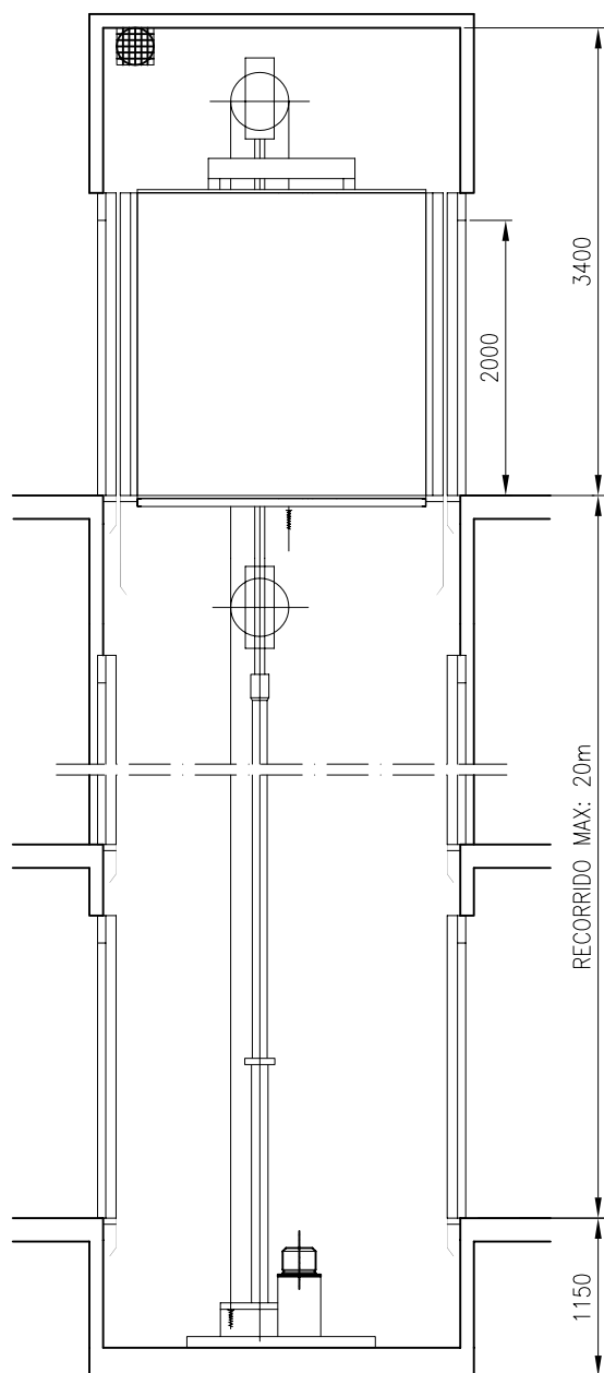
SECCION VERTICAL 1/60
