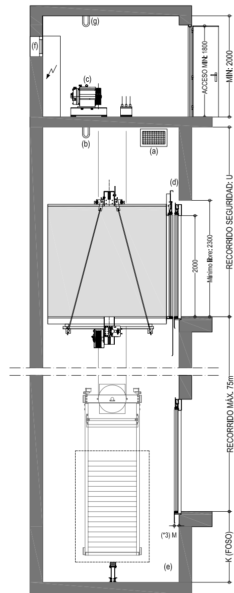
SECCIÓN E.1/75
