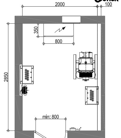
SALA DE MAQUINAS E.1/50
