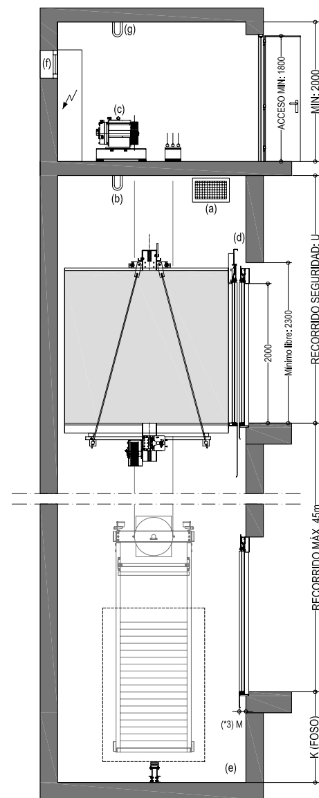
SECCIÓN E.1/75
