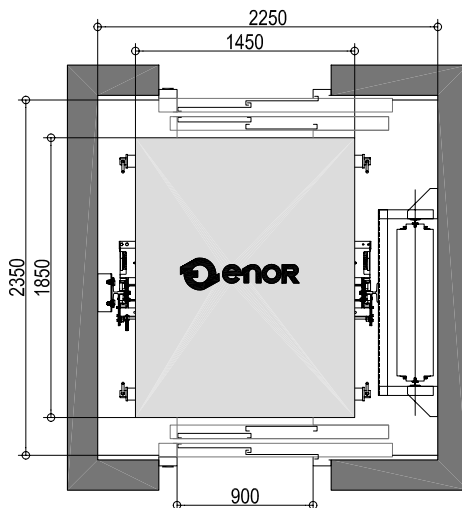
PLANTA GENERAL E.1/50
