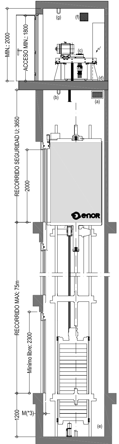
SECCIÓN E.1/60
