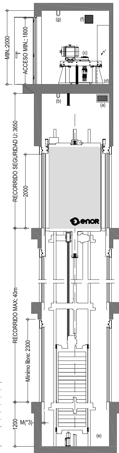
SECCIÓN E.1/60
