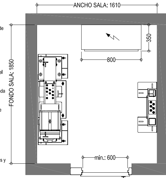
SALA DE MÁQUINAS E.1/30
