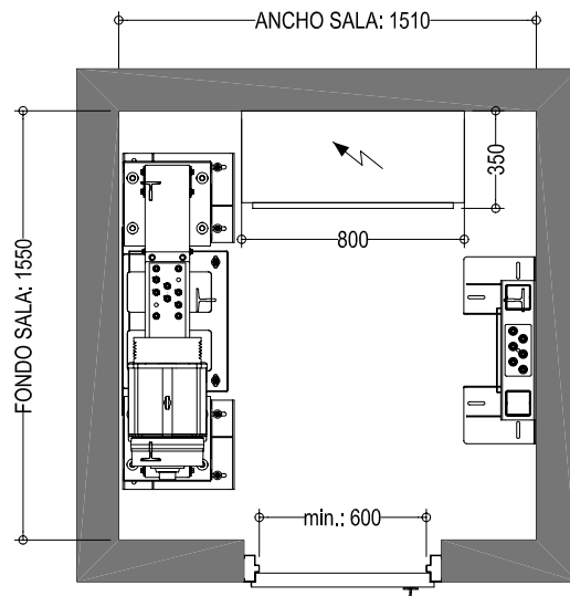
SALA DE MAQUINAS E.1/30
