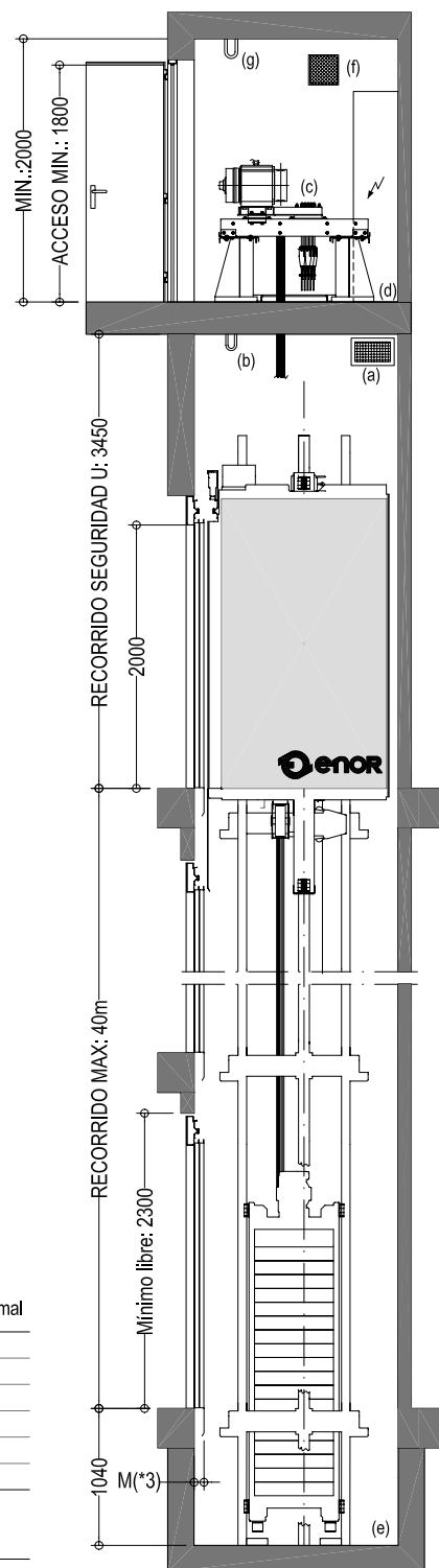
SECCIÓN E.1/60
