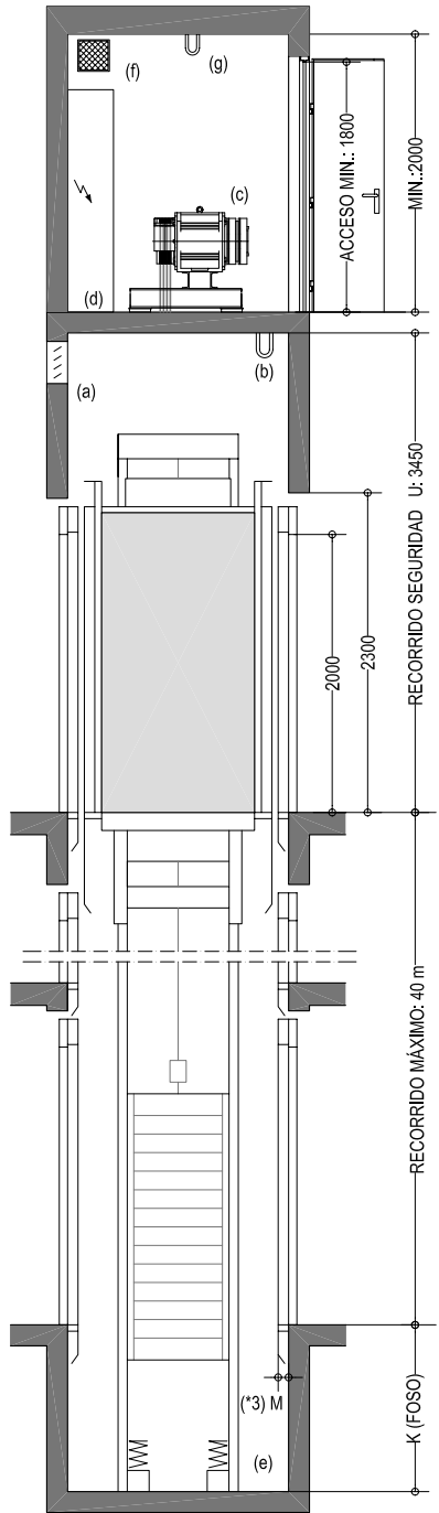
SECCIÓN E.1/60
