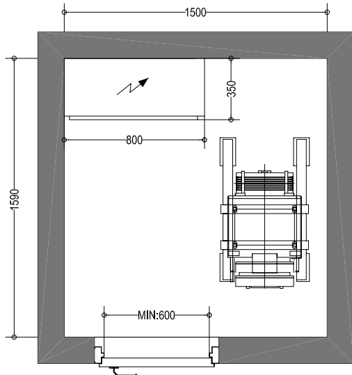
SALA DE MÁQUINAS E.1/30 . Toda la distribución se puede invertir .Apertura de puerta hacia el exterior
