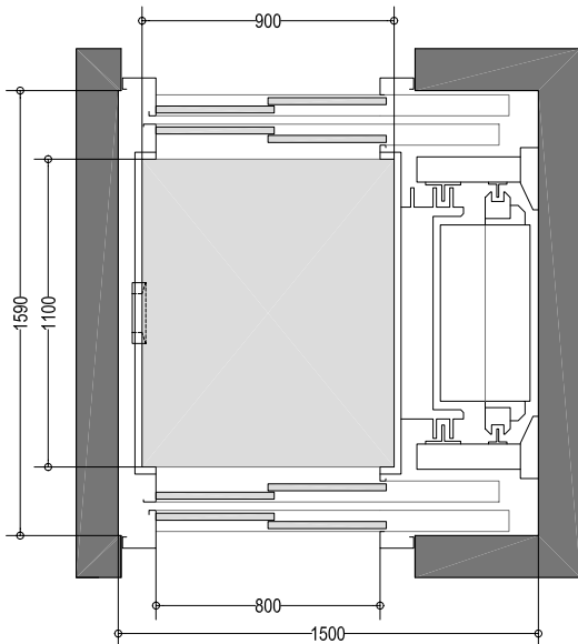
PLANTA GENERAL E.1/30 . Toda la distribución se puede invertir
