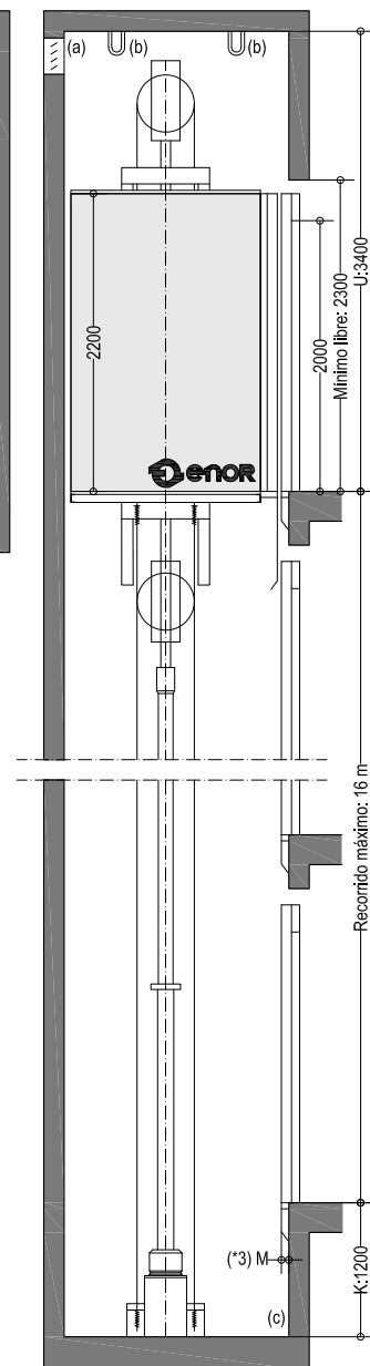
SECCIÓN E.1/60
