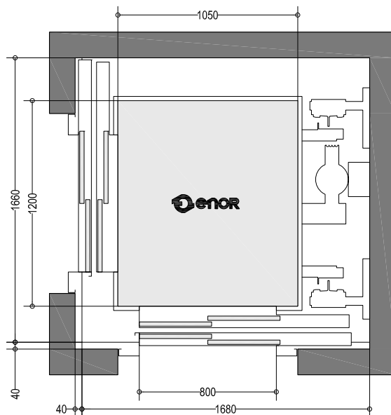
PLANTA GENERAL E.1/30
