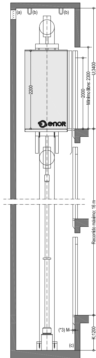
SECCIÓN E.1/60
