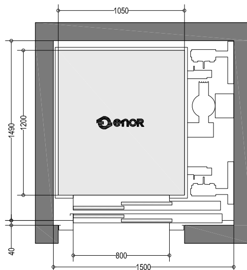
PLANTA GENERAL E.1/30
