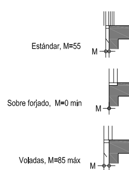
ESQUEMA DISPOSICIÓN PUERTAS DE PISO
