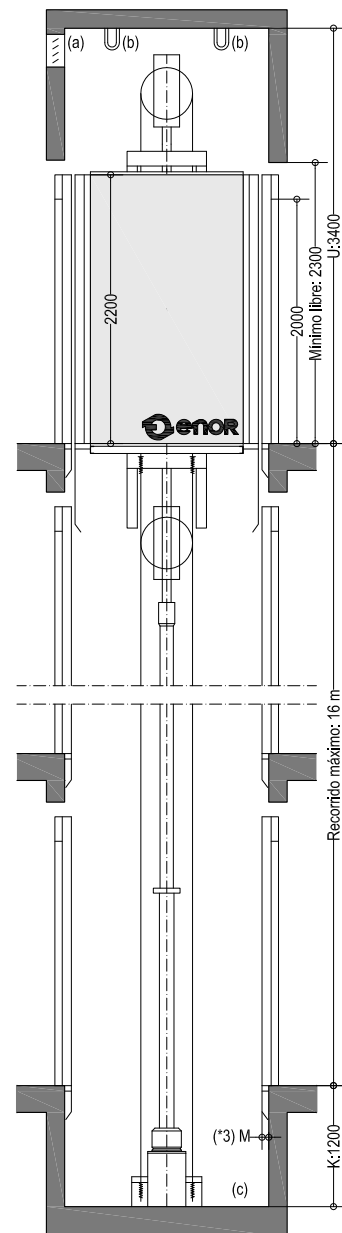
SECCIÓN E.1/60
