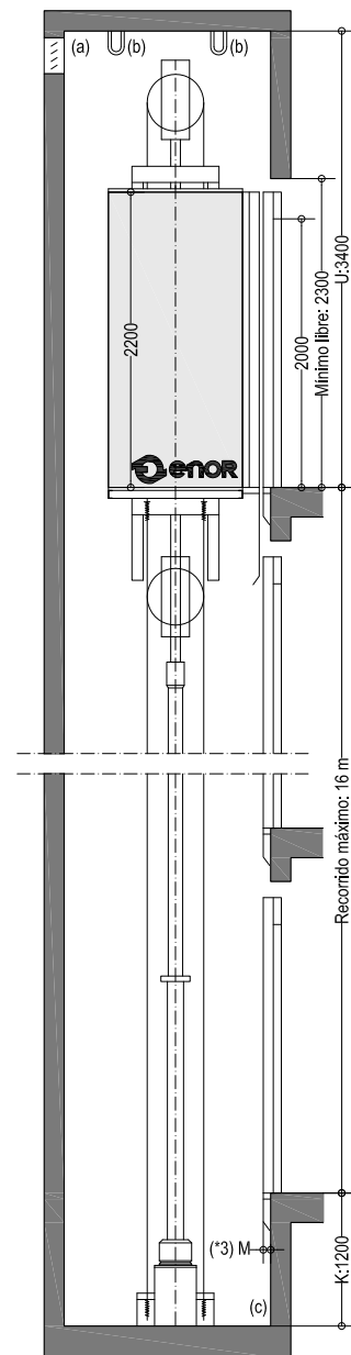
SECCIÓN E.1/60
