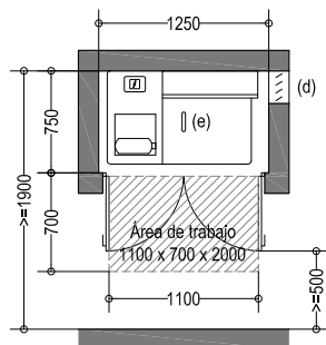
ARMARIO DE MÁQUINAS E.1/60
