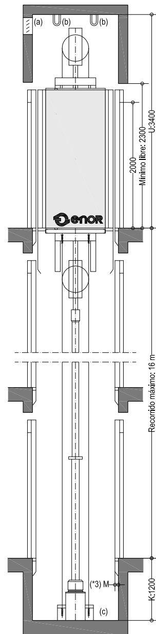
SECCIÓN E.1/60
