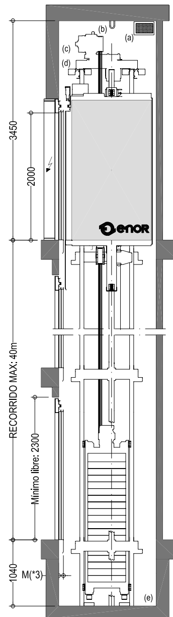
SECCIÓN E.1/60
